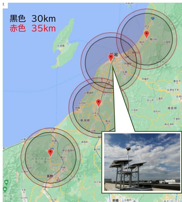
基地局配置図
